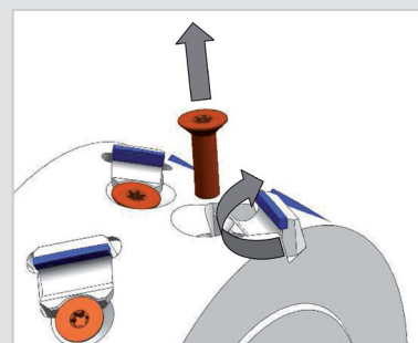
Der Grundkörper des LEUCO DP SmartJointers ist wiederverwendbar. Beschädigte Schneiden können einzeln getauscht werden.
