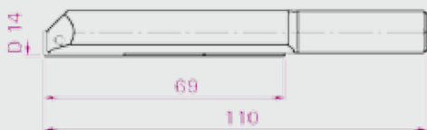
Чертёж LEUCO Концевая фреза со сменными ножами
